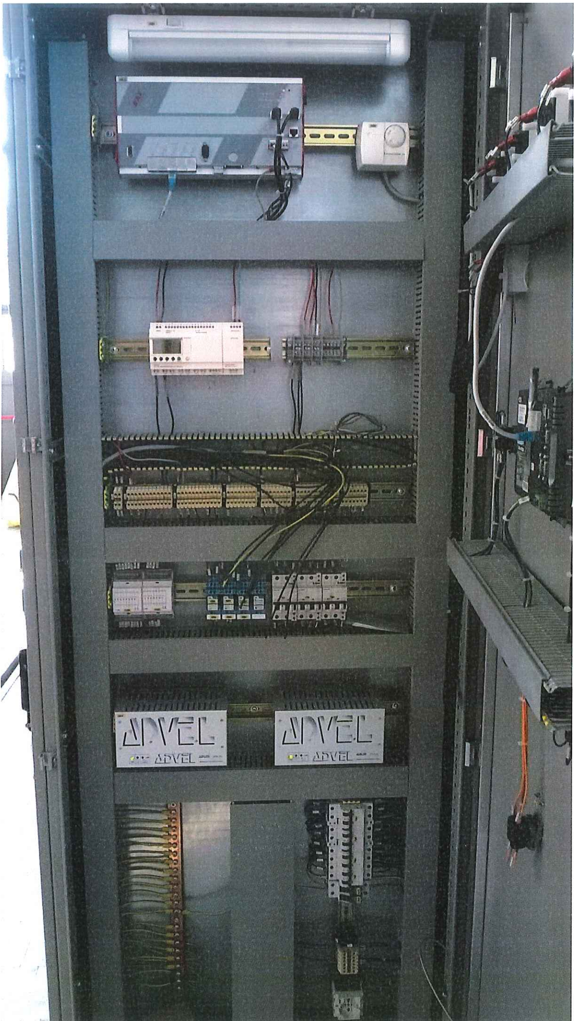
PONT ST. MARTIN - Armadio Regolatore di Velocità Gruppo
